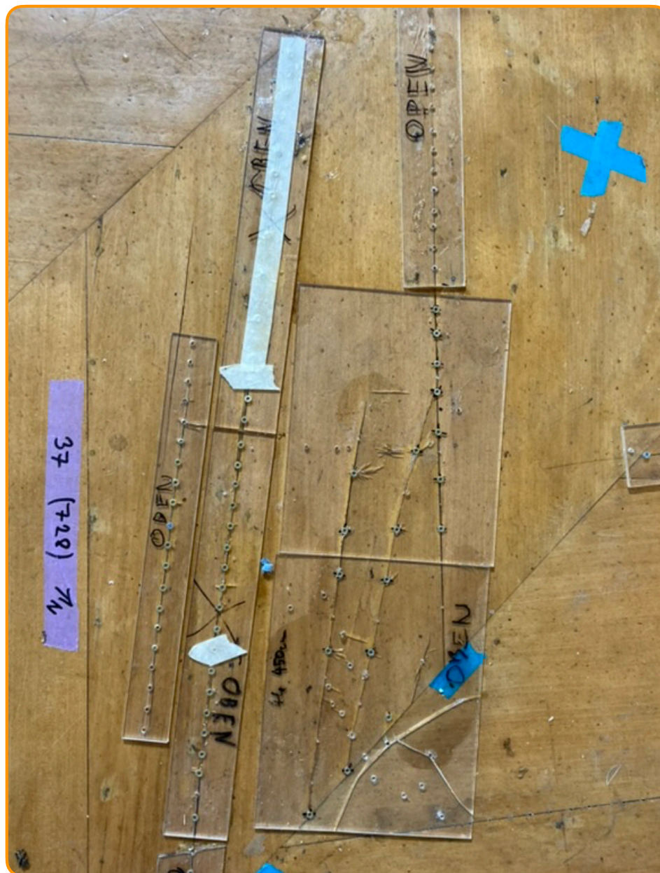
Pomocí plexisklových desek a slabých vrtů
